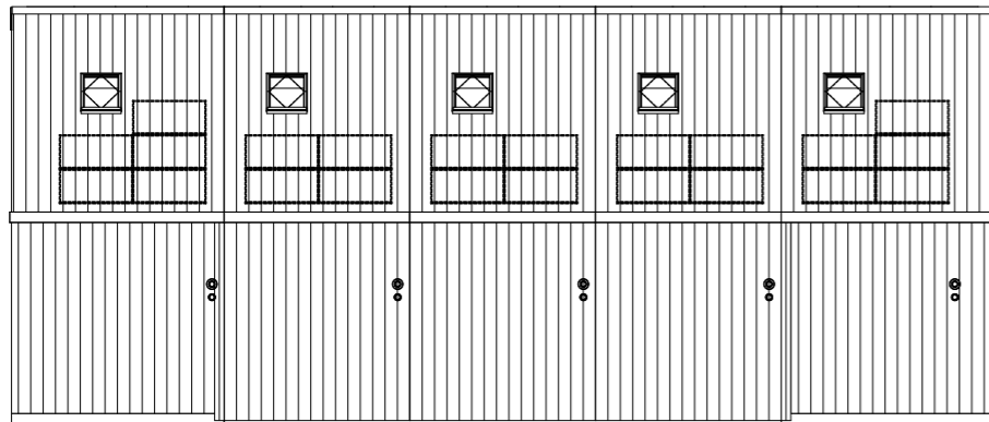
03 dakaanzicht
