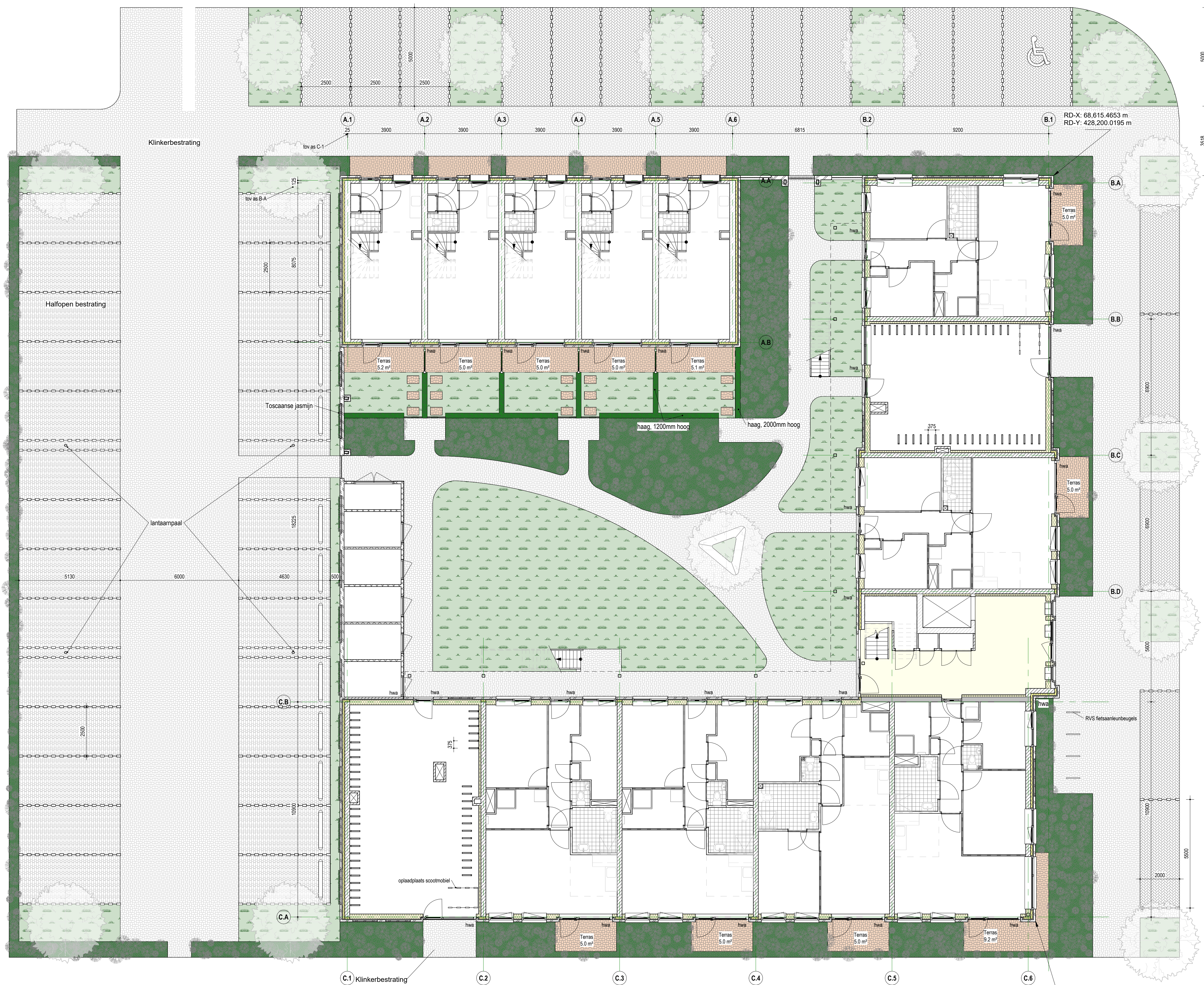
Situatie (tuin, bestrating en parkeerplaatsen)
